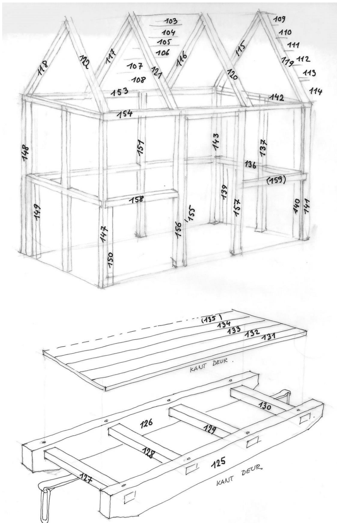
Schets uit het restauratiedossier van de kavane (1990-1991).
