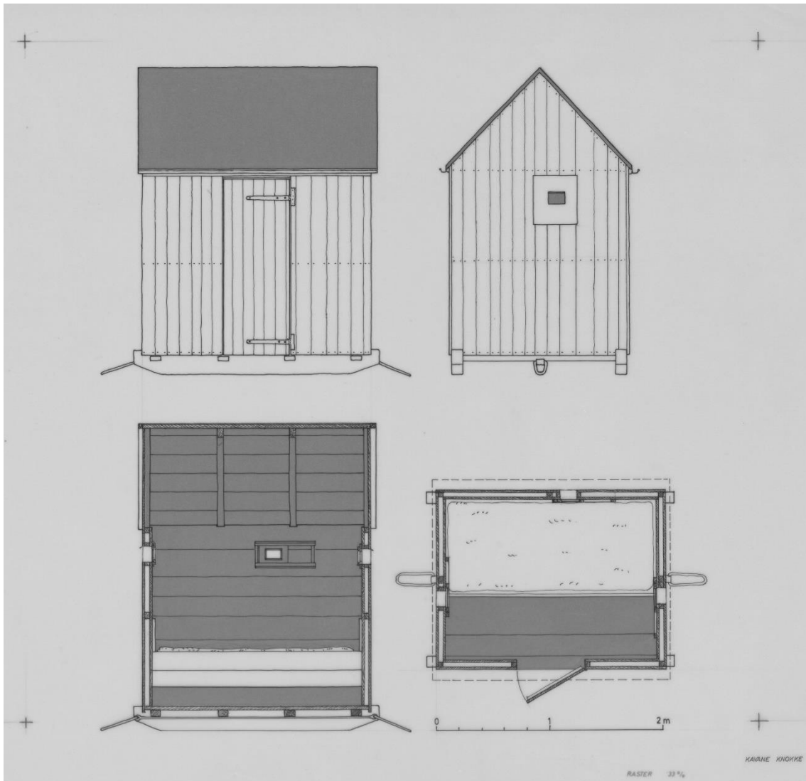
Johan Vansteenkiste maakte in opdracht van de Provincie West-Vlaanderen tekeningen van de kavane (1990-1991).
